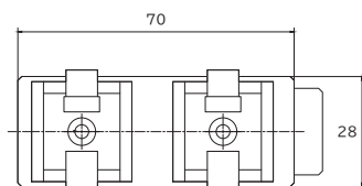
外形図 (単位:mm)
